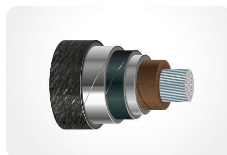
← Cabos com isolamento de papel e óleo
