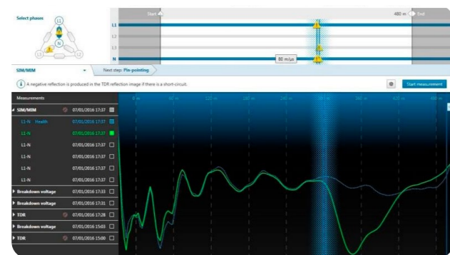
Die Anzeige der BAUR Software 4 ermöglicht eine übersichtliche Darstellung aller wichtigen Einstellungen, Fehlerortungsparameter und der Kabeldaten. Der untere Teil des Bildschirms zeigt die Resultate der Messung und erlaubt eine sofortige Protokollierung wichtiger Ergebnisse.
