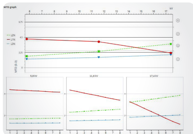
Representação de uma medição de fator de dissipação no relatório ↑
