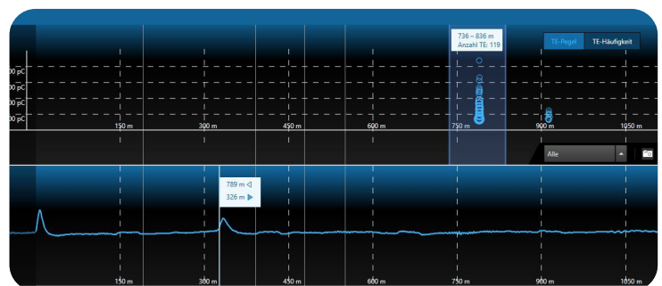
Representação combinada de localização e avaliação de DP ↑
