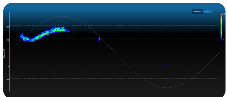
Resolução de fase para um ponto de DP ↑
