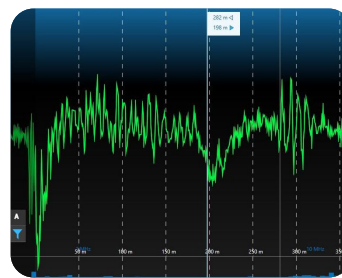
Sinal de DP sobreposto com falhas ↑
