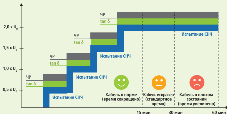
Испытание СНЧ + \tan \delta + ЧР = комплексное испытание MWT
