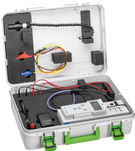
Obrázek: KSG 200 TA (s akumulátorem)
