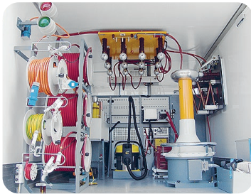
↑ 半自动 transicable 系统, 三相 110 kV
