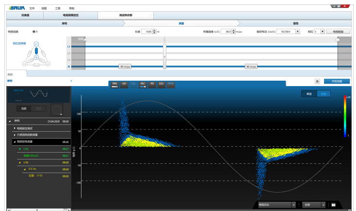
例如: 局部放电测量 – 相位分辨的局部放电图 (PRPD)
