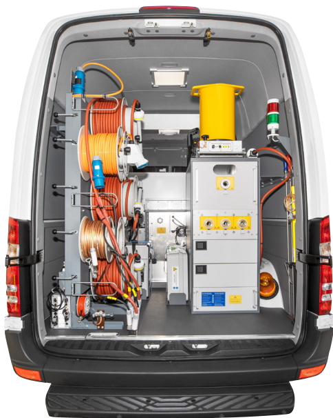
电缆测试车中的 PD-TaD 示例
