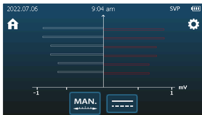
Localisation des défauts de gaine avec tension continue cyclique
