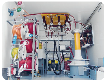
↑ Halbautomatisches transable-System 3phasig, 110 kV
