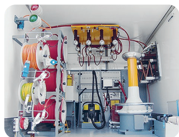
↑ Sistema transcable semiautomático trifásico, 110 kV
