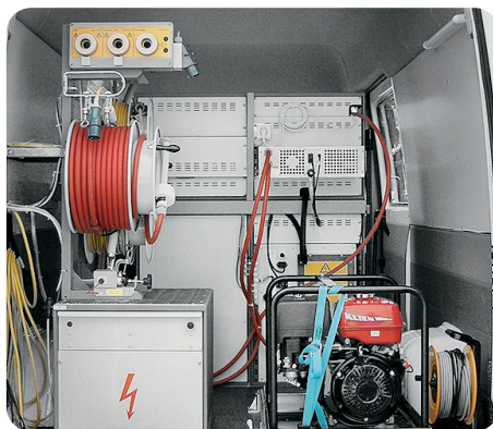
Il sistema transcabile ↑
