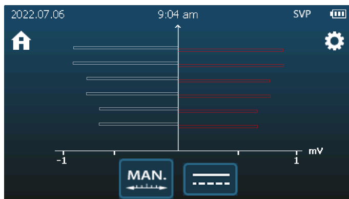
Določanje položaja napake na kabelskem plašču s ciklično enosmerno napetostjo
