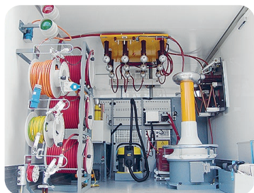
↑ Полуавтоматическая система transcable, трехфазная, 110 кВ
